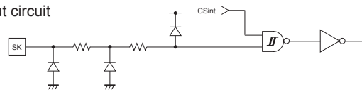
Fig. 49 Input circuit (SK)
